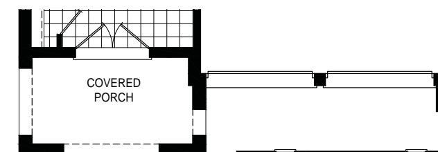
ELEV. C
